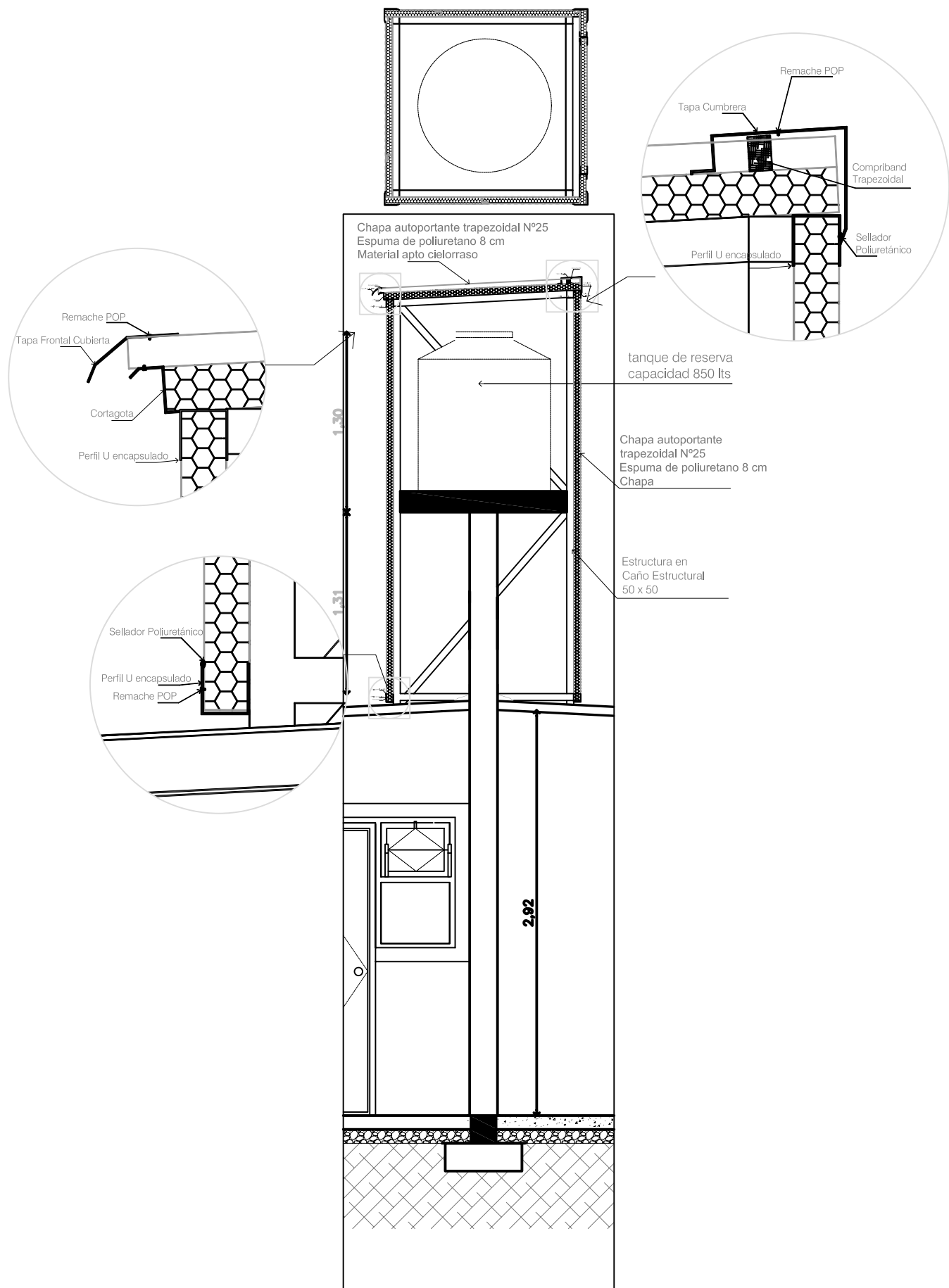
Corte A-A
